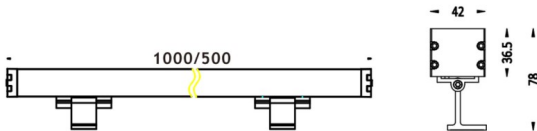
Esquema
