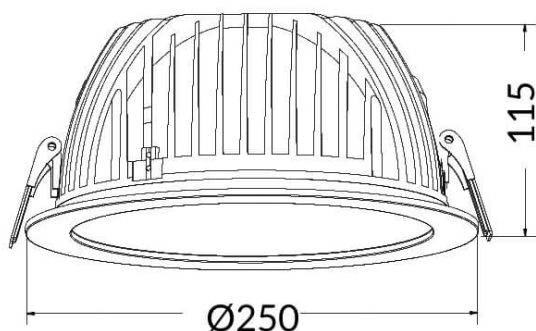
Dessin technique
